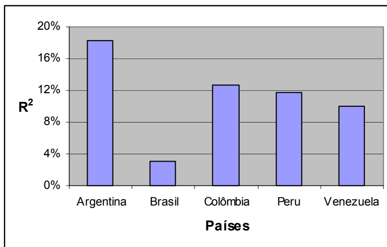
Gráfico 1 – R 2 Ajustado
