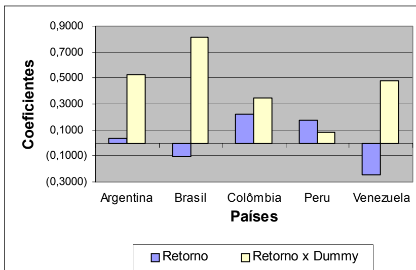
Gráfico 2 – Comportamento dos Coeficientes da Regressão
