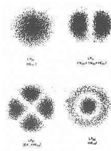
Figura 6 - Padrões de Modos guiados em Fibras Ópticas
