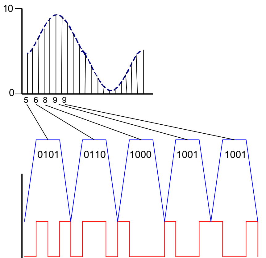
Figura 16 - Digitalização do canal analógico
