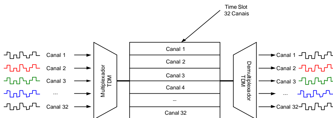
Figura 17 - Multiplexação por divisão do tempo - TDM
